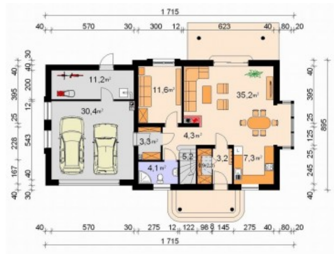
RZUT PARTERU
