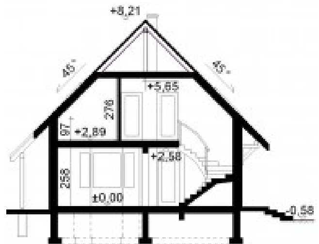
Przekrój A-A
